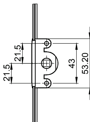
DETALLE A ESCALA 1 : 2
